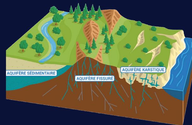
Des aquifères de nature différente (OFB, Matthieu Nivese (d'après OIEau), 2018)
